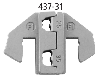
Embout Caméléon pour connecteur virole (F1) (Ca 2 à 4)
